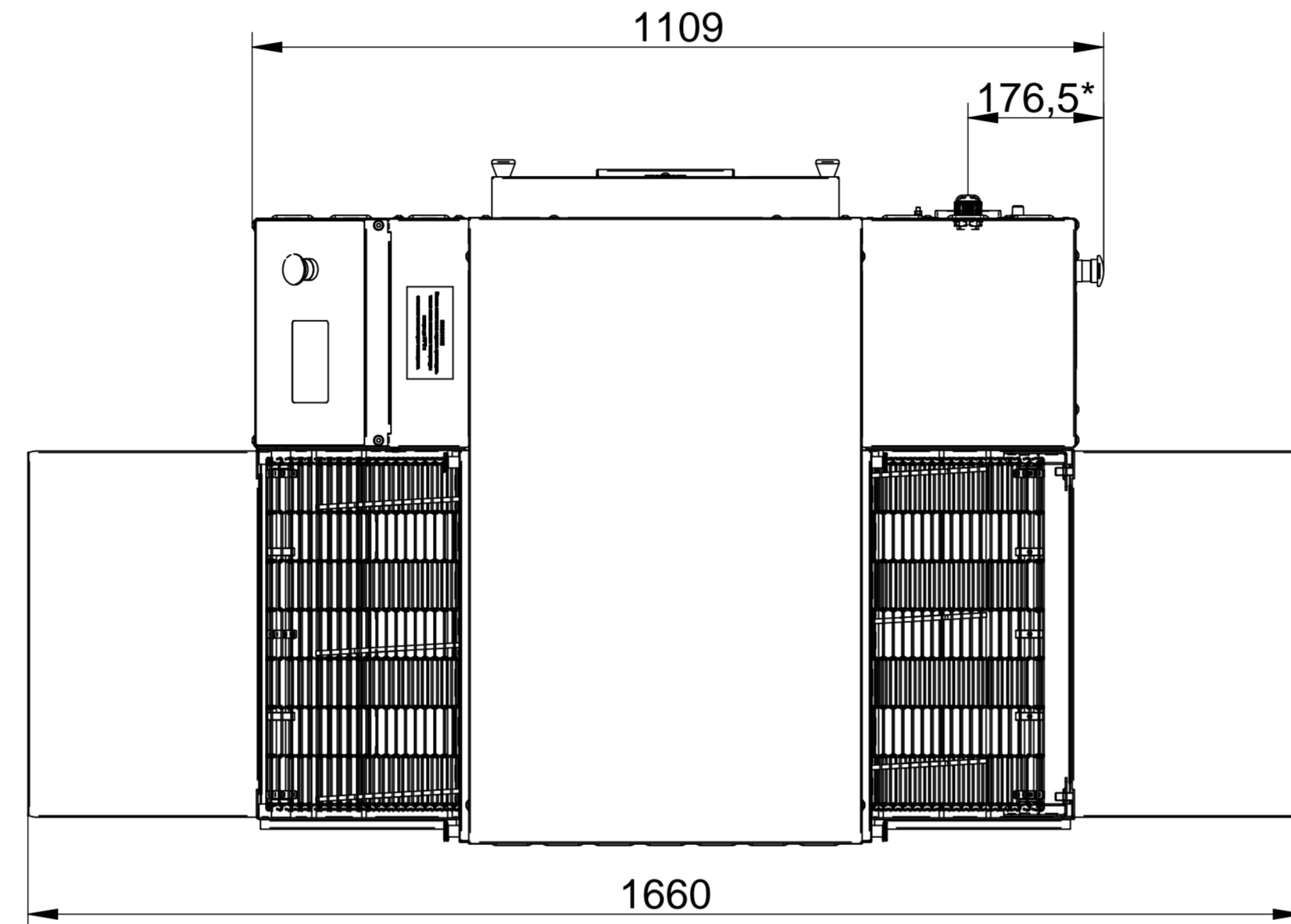
ПЭК-400П 21000003142
